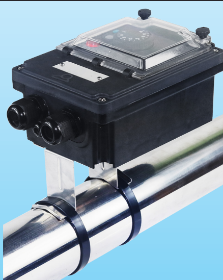
Esempio di montaggio con opzione di staffa di montaggio posteriore 6YTPT su tubo verticale
